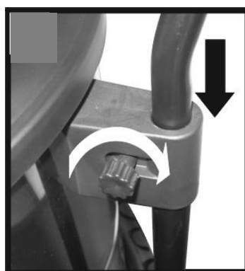
Figura 6 – Montaggio manubrio
