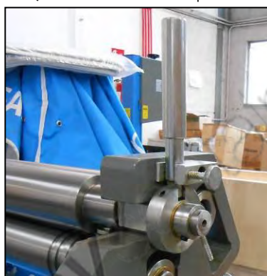
Figura 14 - Fermo del rullo mobile.
