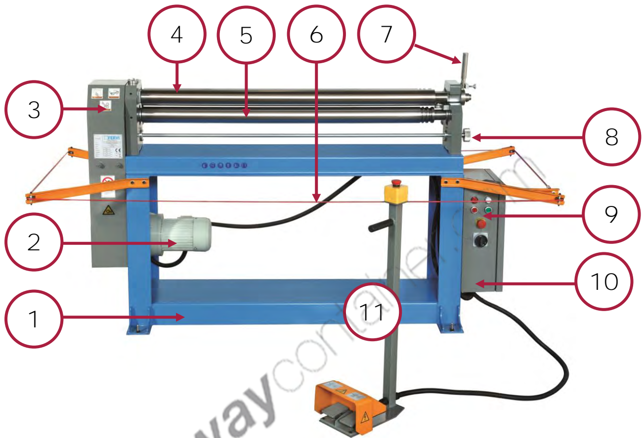
Figura 1 – Vista generale.
