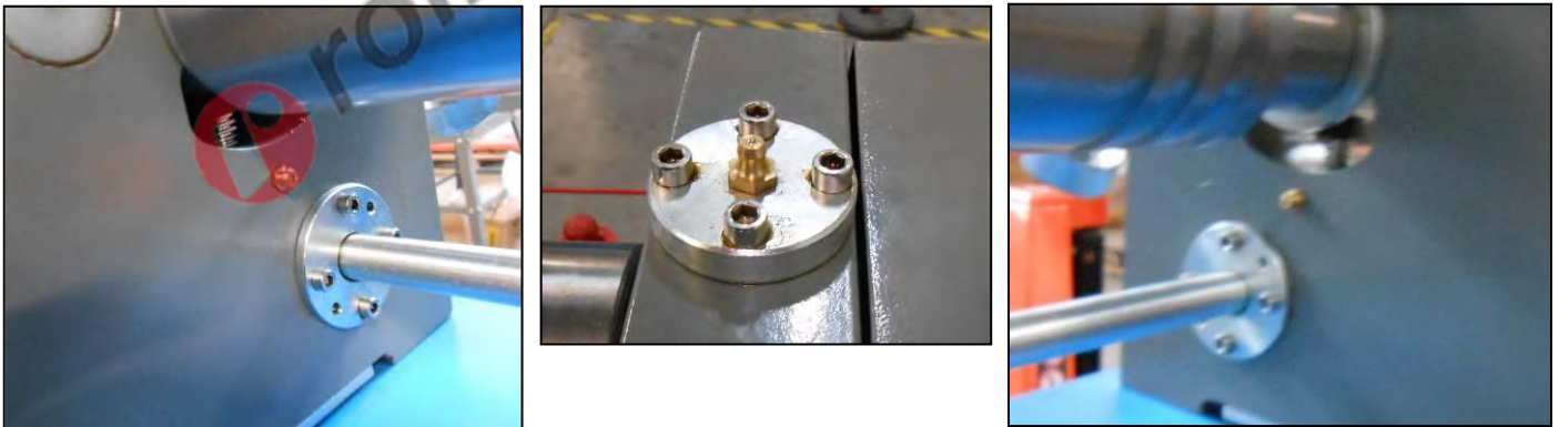
Figura 23 – Posizioni di ingrassaggio.
