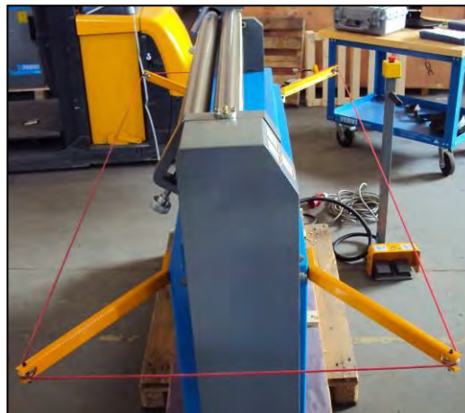
Figura 5 – Riparo degli ingranaggi.
