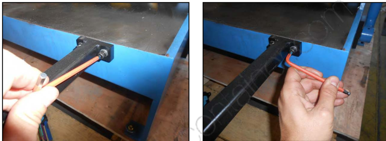
Figura 4 – Montaggio dei supporti anteriori della lamiera.
