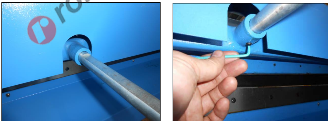
Figura 5 – montaggio dei supporti della battuta posteriore.
