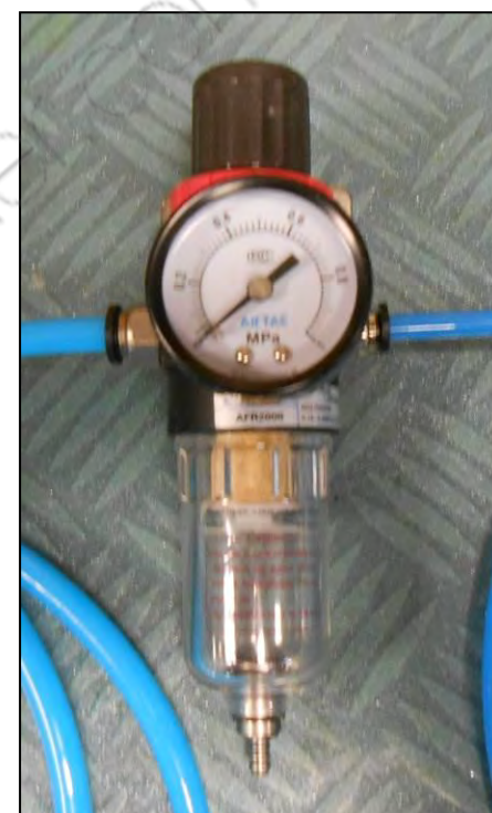
Figura 11 – Collegamento aria compressa.
