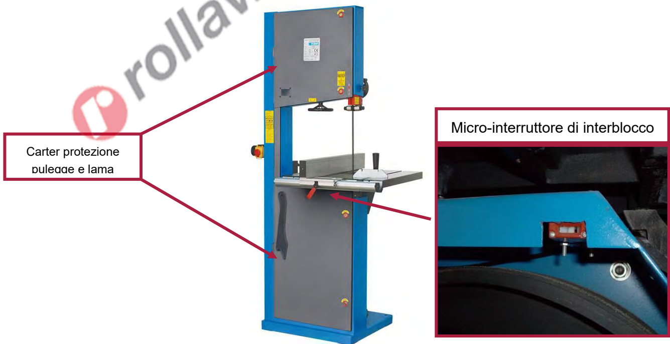
Figura 17 – Interblocco del riparo.
