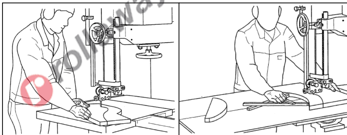
Figura 36 – Esecuzione di tagli curvi o irregolari.
