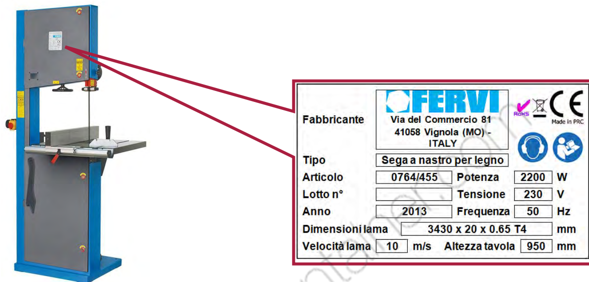
Figura 3 - Targhetta di identificazione.
