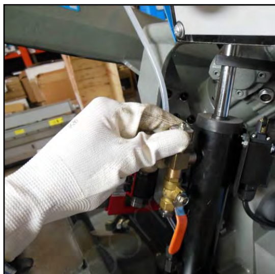
Figura 34 – Regolazione velocità.
