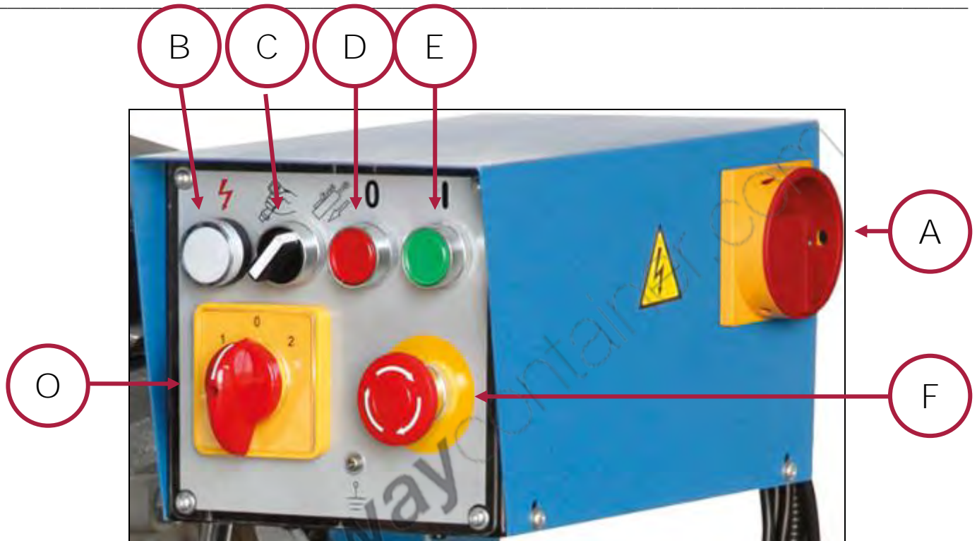
Figura 3 – Dettaglio quadro comandi.
