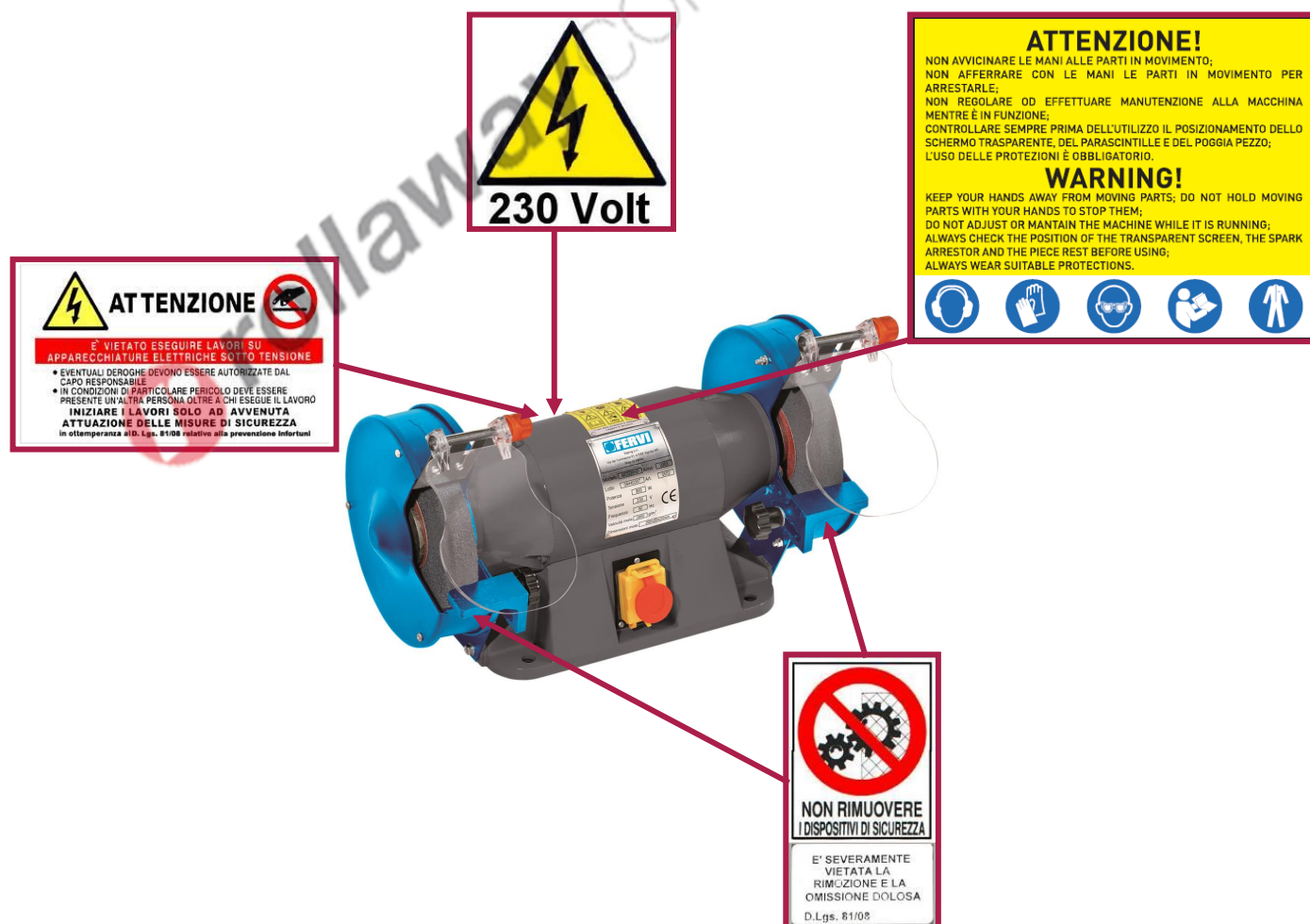
Figura 3 – Pittogrammi di segnalazione ed attenzione.
