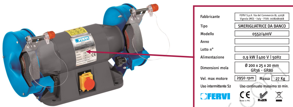
Figura 2 – Targhetta di identificazione.
