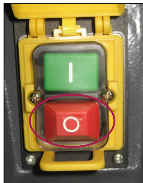
Figura 12 – Pulsante di stop.
