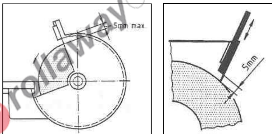
Figura 6 – Regolazione degli schermi di protezione.
