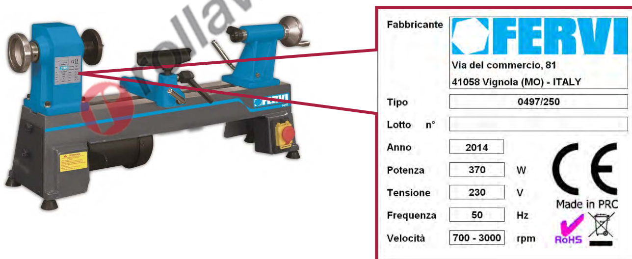
Figura 7 – Targhetta di identificazione Art. 0497/250.
