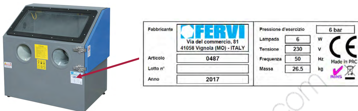
Figura 2 - Targhette di identificazione.
