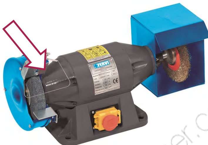
Figura 5 – Dettaglio schermi di protezione.
