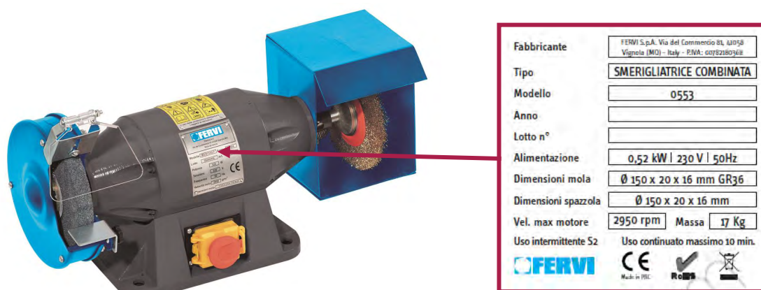
Figura 2 – Targhetta di identificazione
