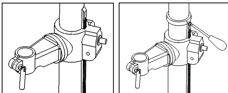
Figura 3 - Installazione supporto tavola
