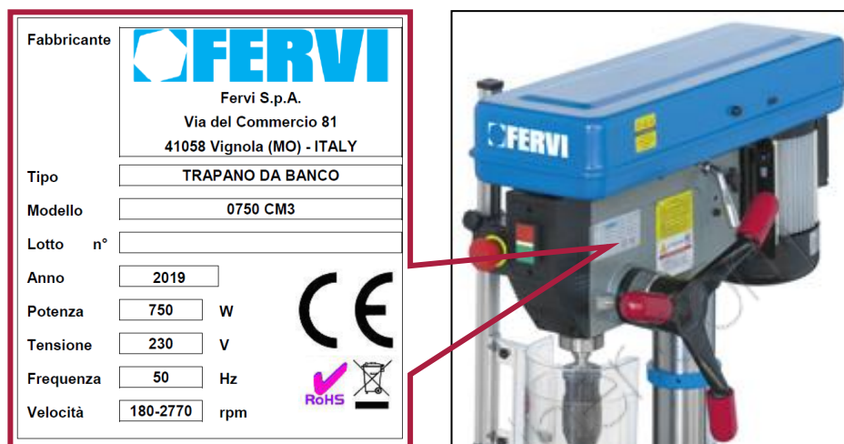
Figura 20 – Targhetta di identificazione.
