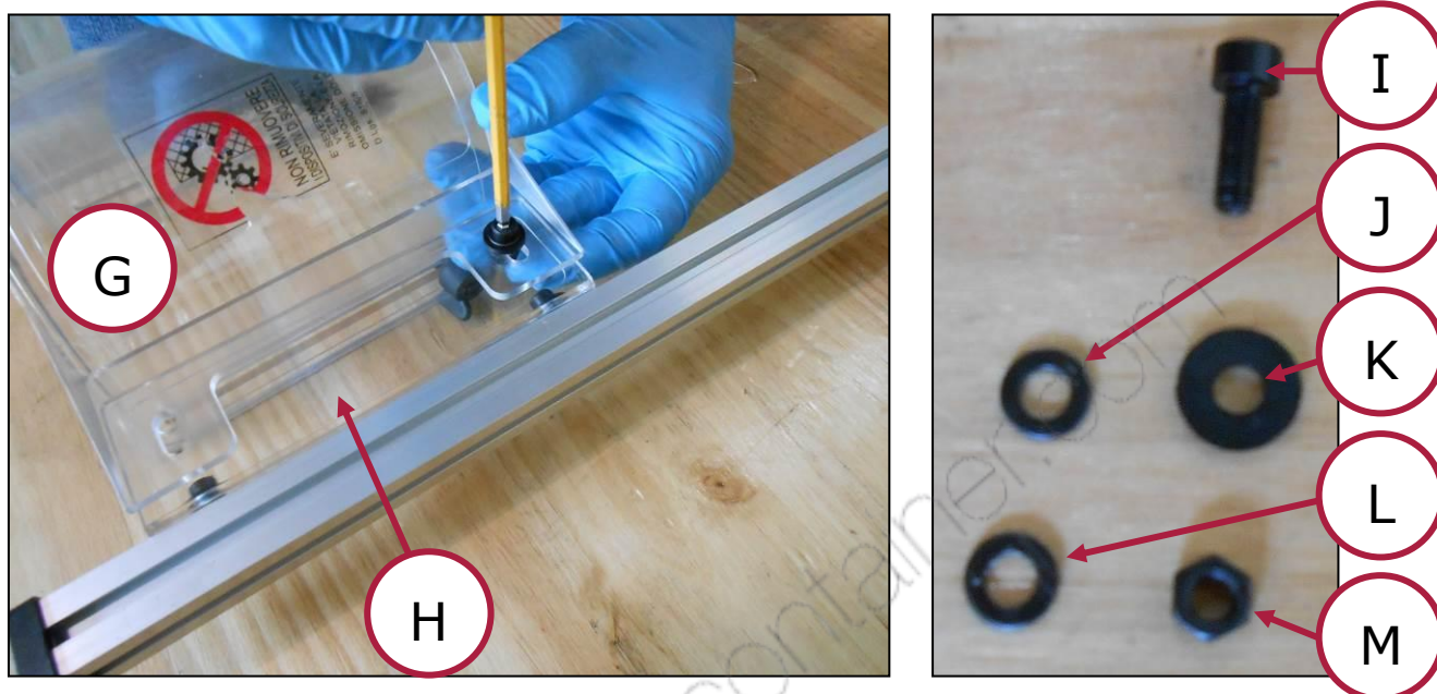
Figura 15 – Montaggio riparo
