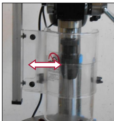
Figura 34 - Scorrimenti del riparo in senso verticale e longitudinale
