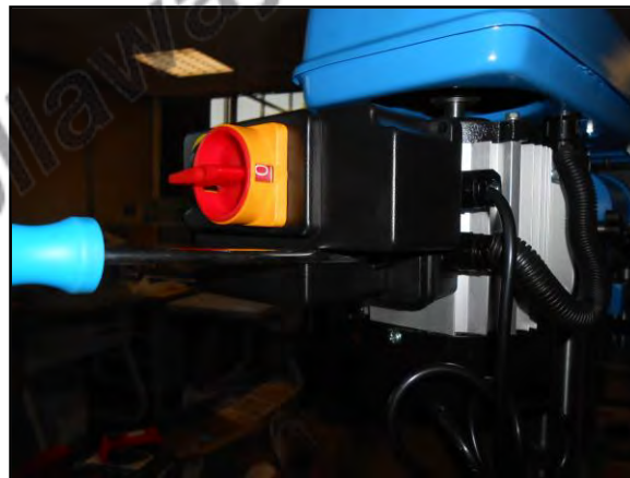
Figura 10 – Montaggio della scatola elettrica.
