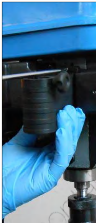
Figura 5 – Montaggio del blocco microinterruttore
