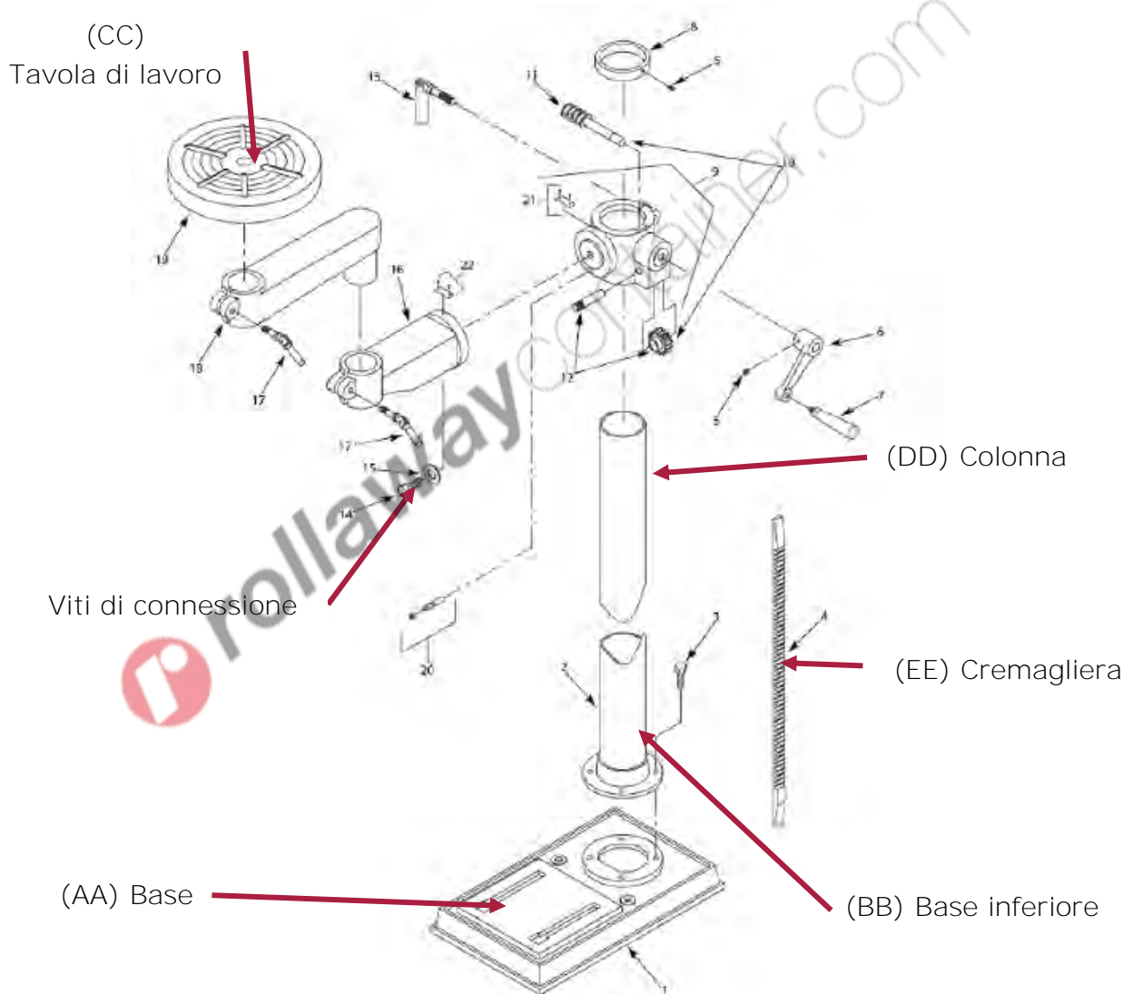
Figura 1 – Componenti per l'assemblaggio della macchina.
