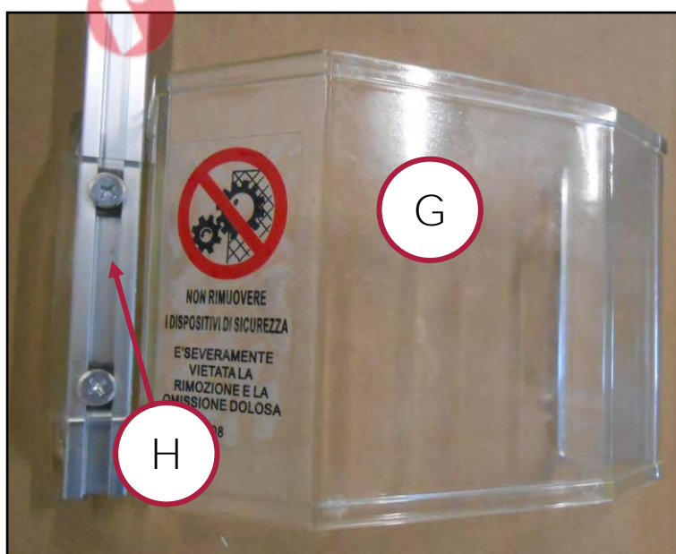
Figura 6 – Montaggio riparo
