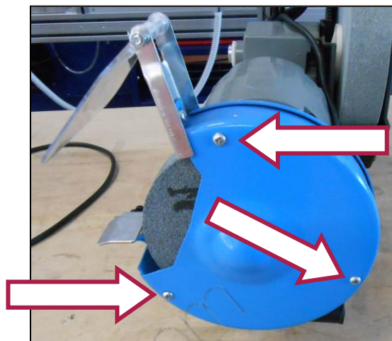
Figura 14 – Carter di protezione.
