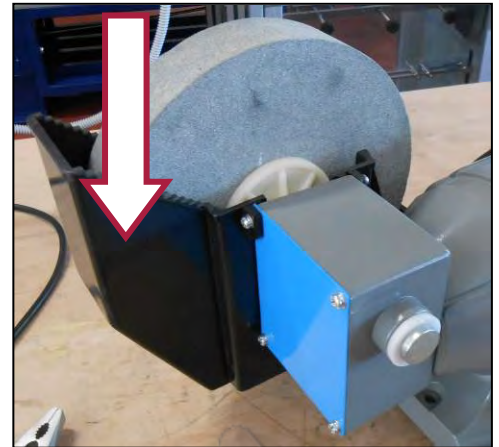
Figura 13 – Dettaglio mola ad acqua e gradini.
