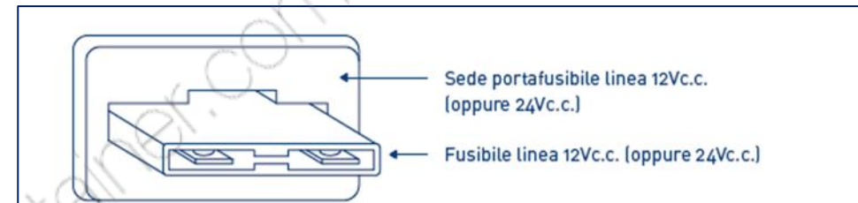
Disegno 4: Fusibile linea tensione continua 12Vc.c. (24Vc.c.)
