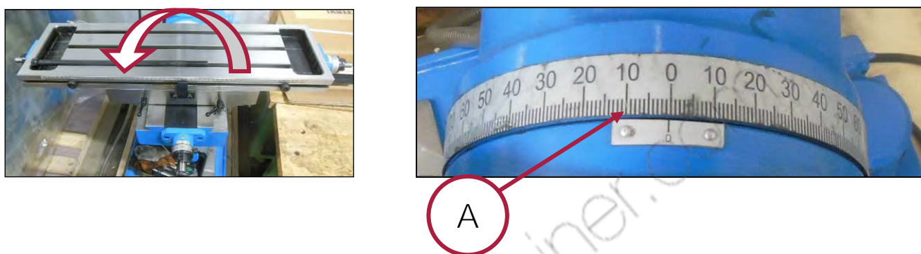
Figura 12 – Tavola di lavoro e scala graduata.
