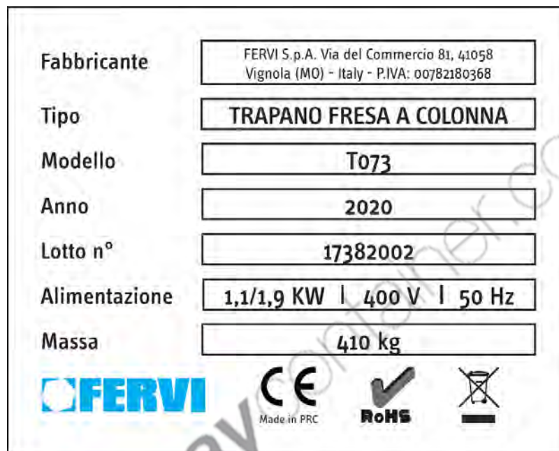
Figura 2 – Targhette CE delle macchine.
