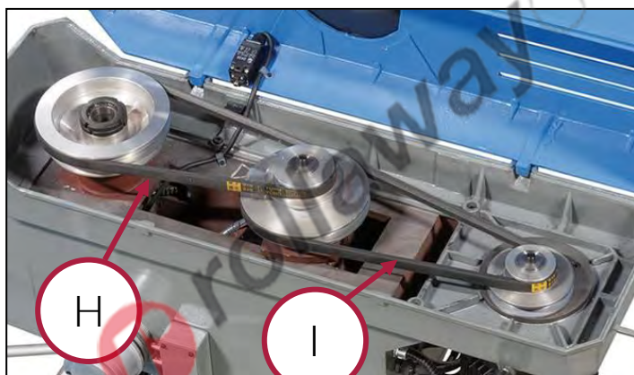
Figura 7 – Regolazione velocità.
