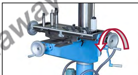
Figura 13 –Volantino avanzamento trasversale.
