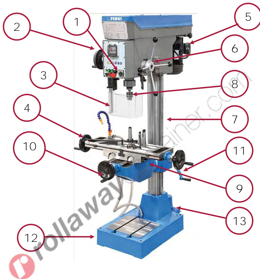
Figura 1 – Elementi principali.
